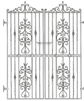
GD-1 (W1600×H2000)
